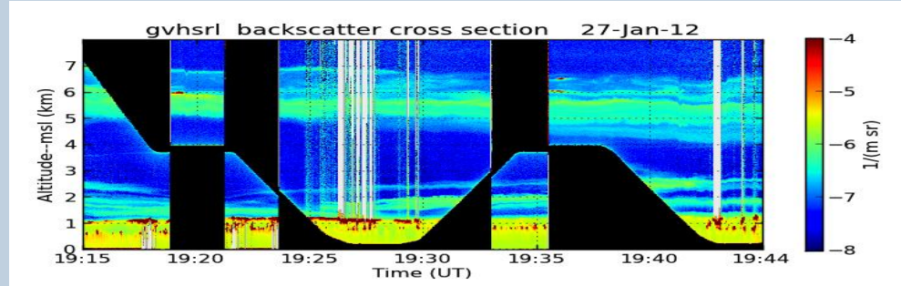
HSRL backscatter, TOREDO, 2012/01/12
